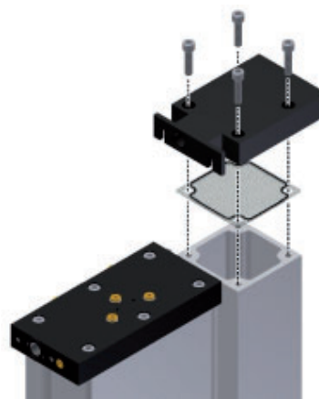
Allentare la piastra di testa
