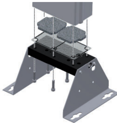
Allentare la piastra delle valvole magnetiche
