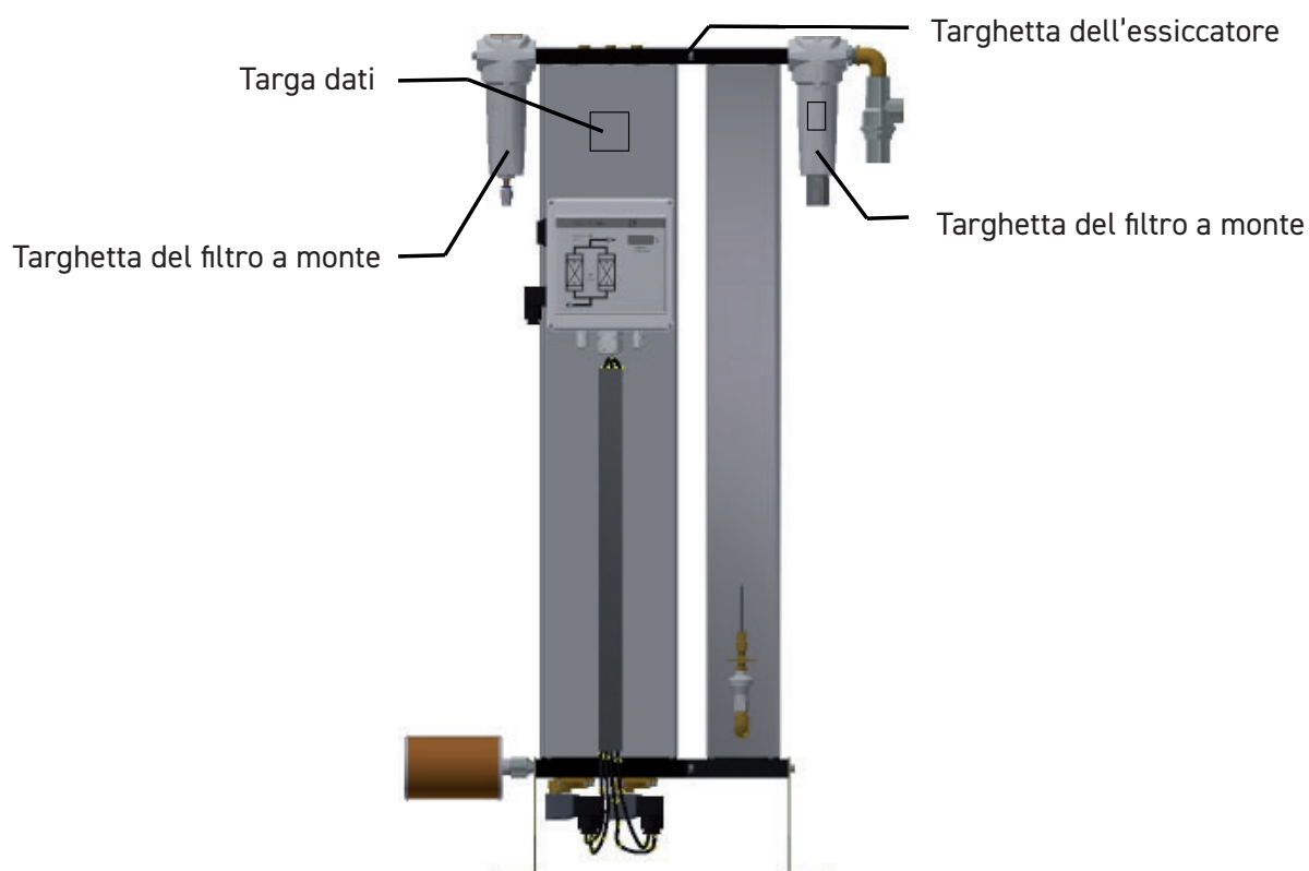
Vista frontale
